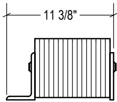
P1 CONFIG.
