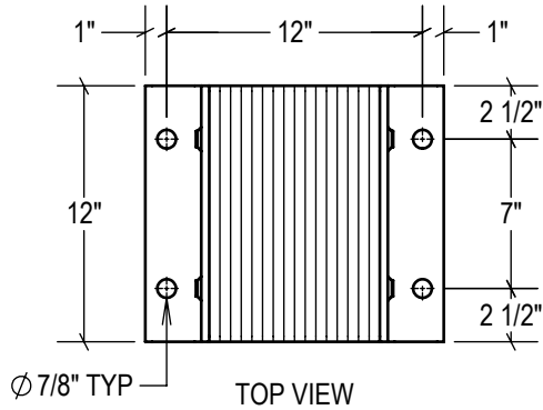
P2 CONFIG.
