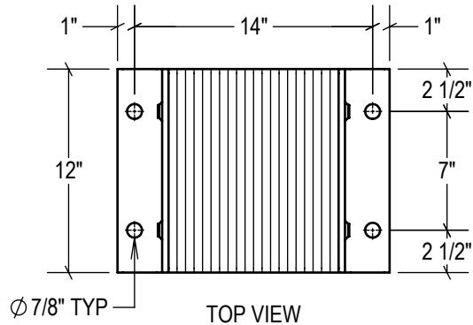
P2 CONFIG.
